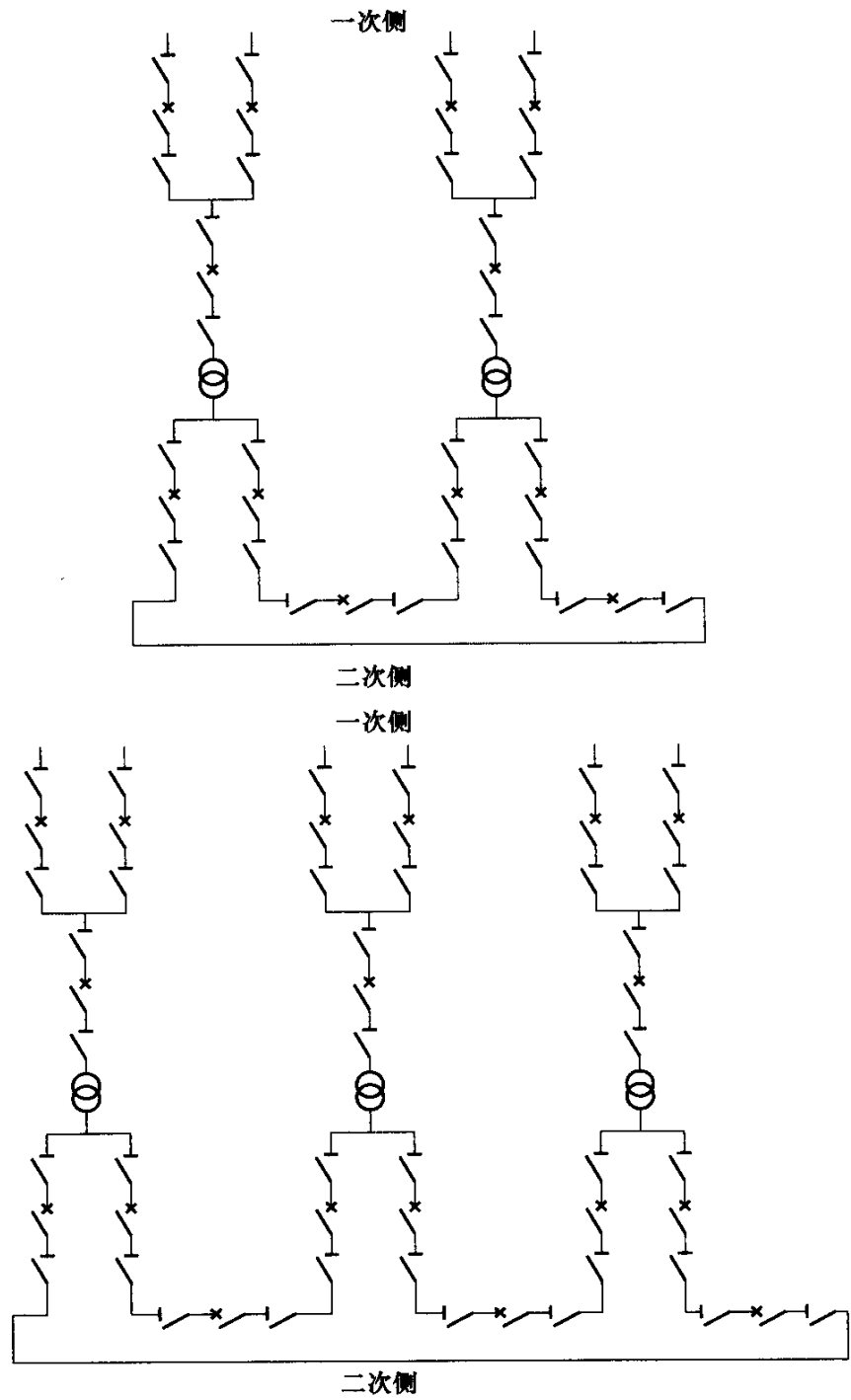
图 D.0.5 环入环出
