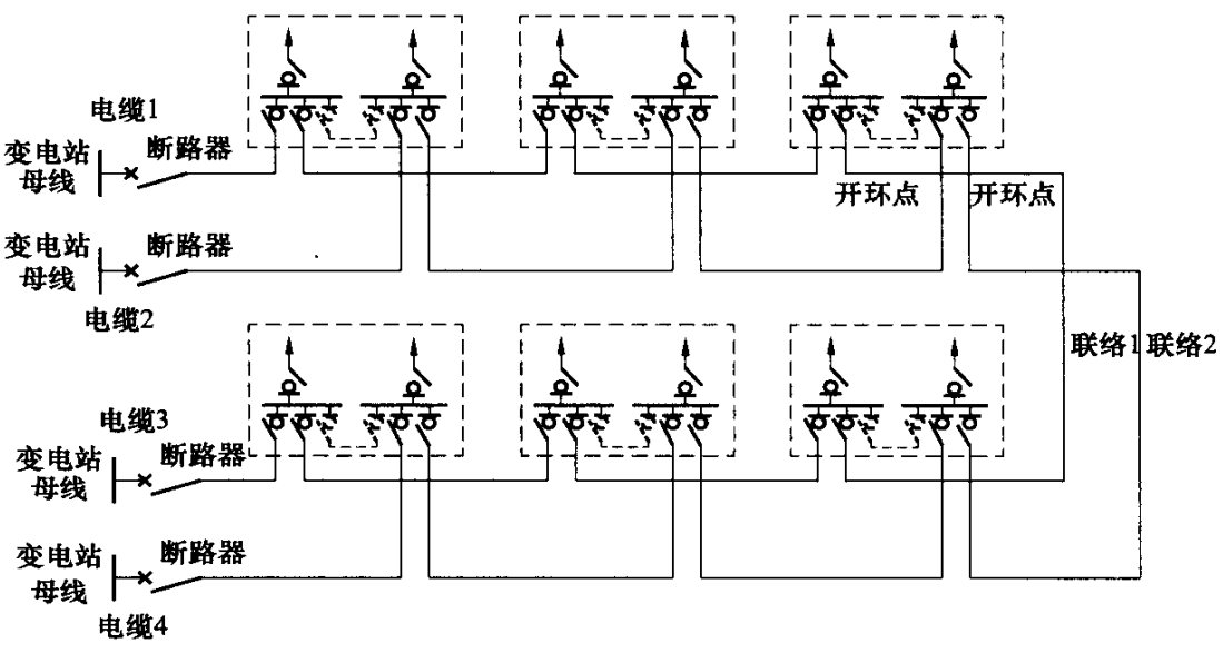
图 B.0.2-2 双环式
