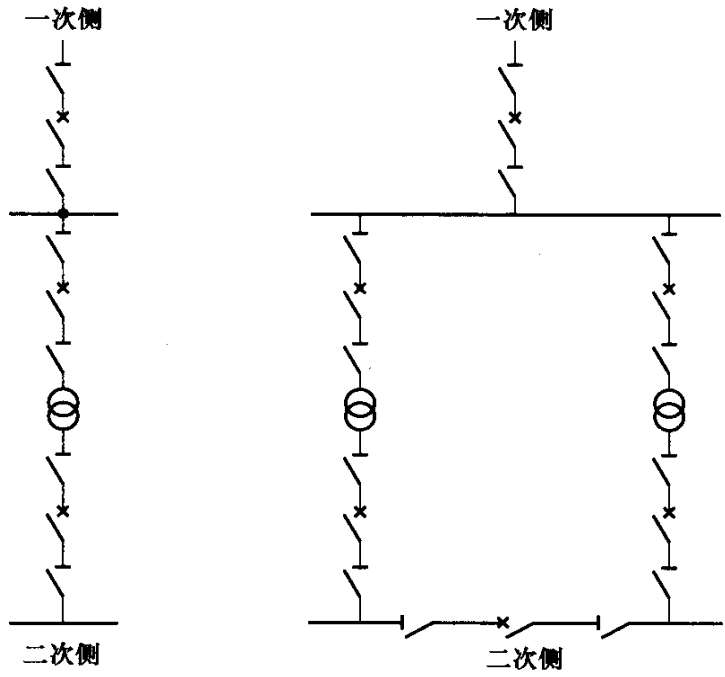
图 D.0.1 单母线
