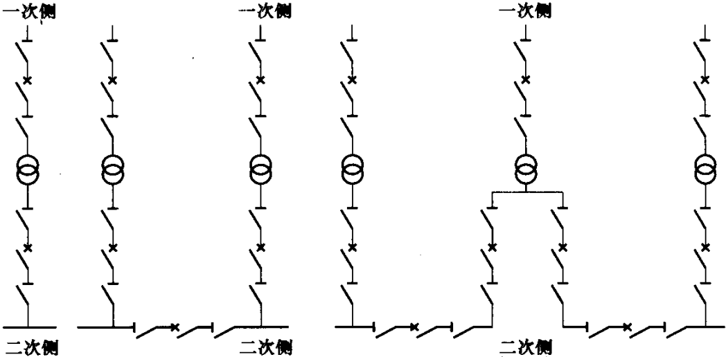
图 D.0.4 线路变压器组
